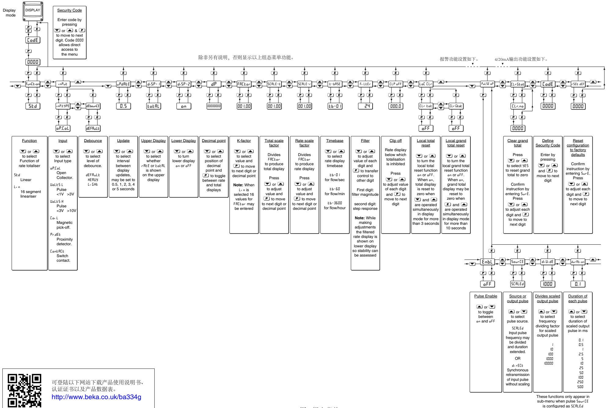
图 5 组态菜单
