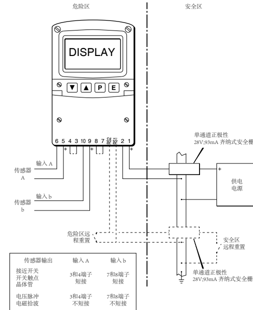
图3 典型计时器回路
