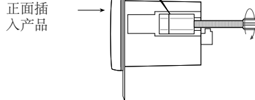
图2 安装步骤
