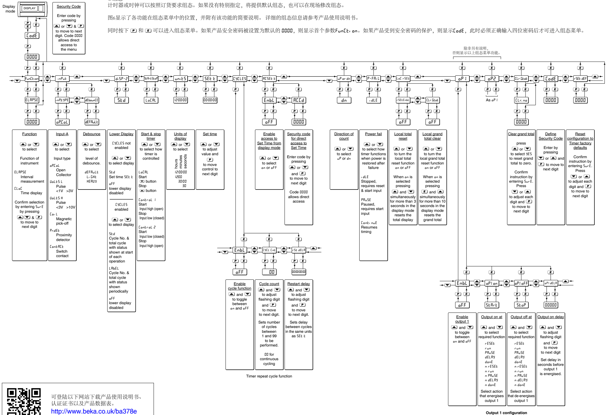
图 6 组态菜单
